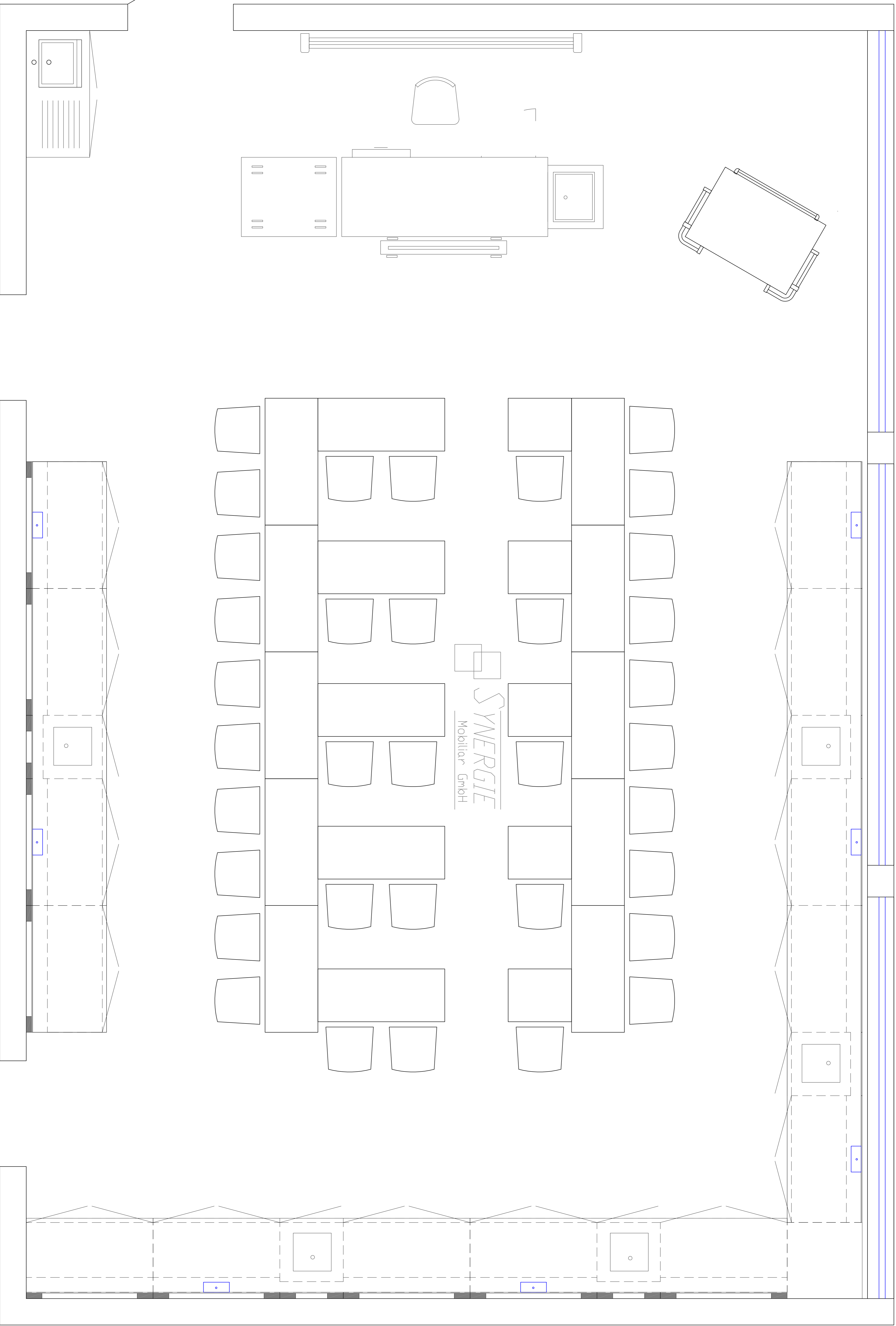
Schüler-Wandexperimentierplätze mit Medienversorgung und beweglichen Tischen mittig
